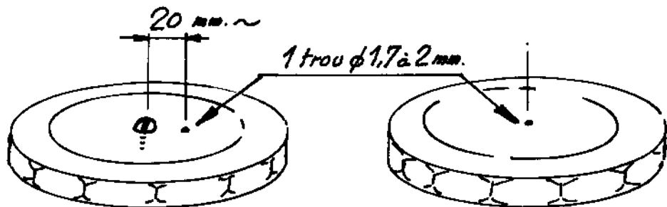
Bouchon plastique comportant 1 vis PARKER
