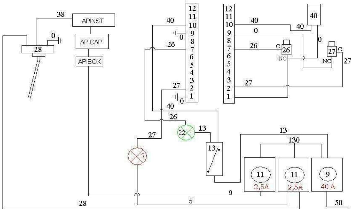
CABLAGE CIRCUIT CARBURANT APM30
