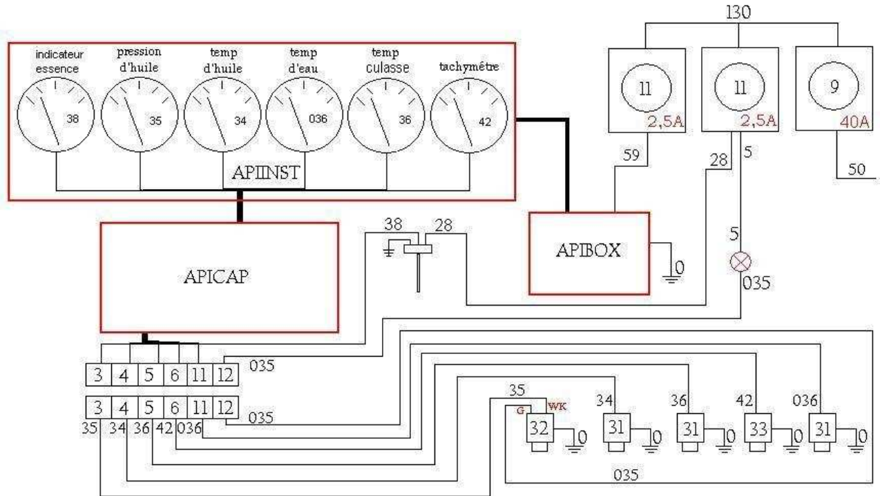
CABLAGE CONTROLE MOTEUR JAUGEUR ESSENCE APM 30
